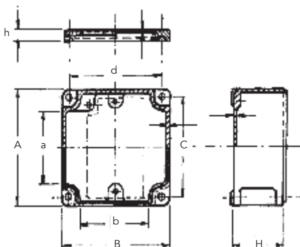
DIMENSIONI TIPO AJB...SS SPESSORE 9 mm
